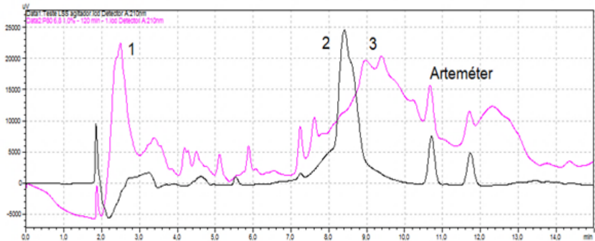
Figura 34 - Comparação dos cromatogramas para os meios pH 6,8 + 1,0% de P80 (p/v) e pH 6,8 + 1,0% de LSS (p/v), picos 1-3 representam a lumefantrina
