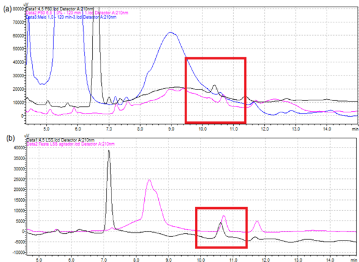
Figura 36 - Comparação dos cromatogramas diferentes meios: a) 1,0% de P80 (p/v) nos pH 1,2, 4,5 e 6,8; b) 1,0% de LSS (p/v) nos pH 4,5 e 6,8
