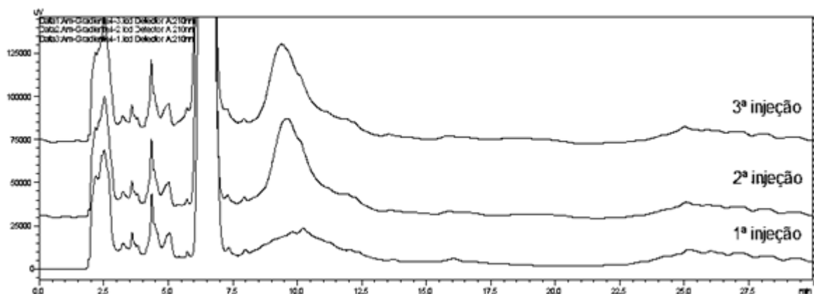
Figura 22 - Cromatogramas de três injeções do Gradiente 4, obtidas em coluna Symmetry®, fluxo de 1,0 mL/min, em uma mesma sequência
