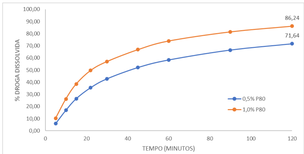
Figura 31 - Perfil de dissolução de lumefantrina em meio de dissolução pH 1,2 + 0,5% de P80 (p/v) e pH 1,2 + 1,0% de P80 (p/v), pás, 100 rpm
