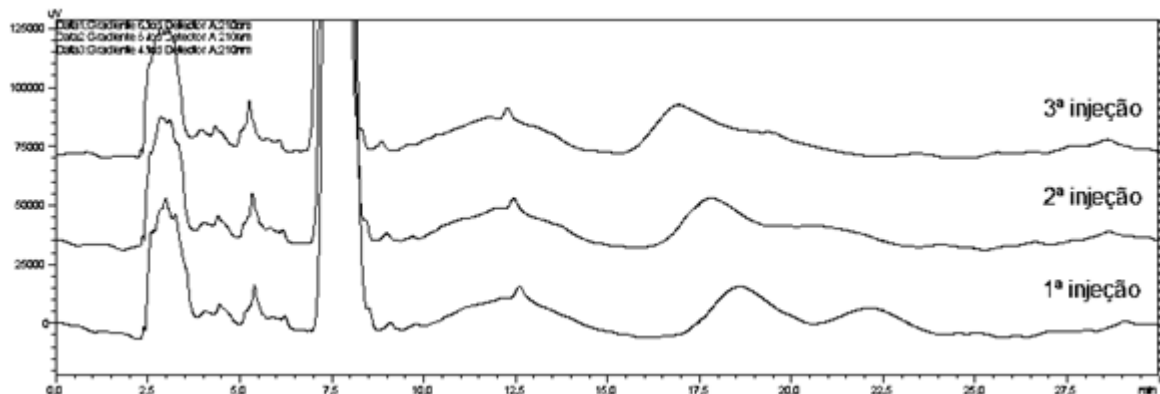
Figura 21 - Cromatogramas de três injeções do Gradiente 2, obtidas em coluna Symmetry®, fluxo de 1,0 mL/min, em uma mesma sequência
