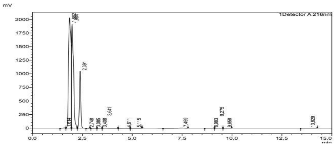
Figura 11 - Cromatograma obtido em coluna Symmetry®, FM composta por ACN:ácido trifluoroacético 0,05% (v/v) (80:20 %v/v), fluxo de 1,2 mL/min
