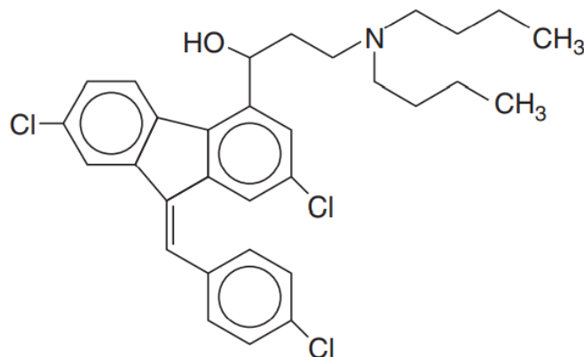
Figura 4 – Estrutura química da lumefantrina
