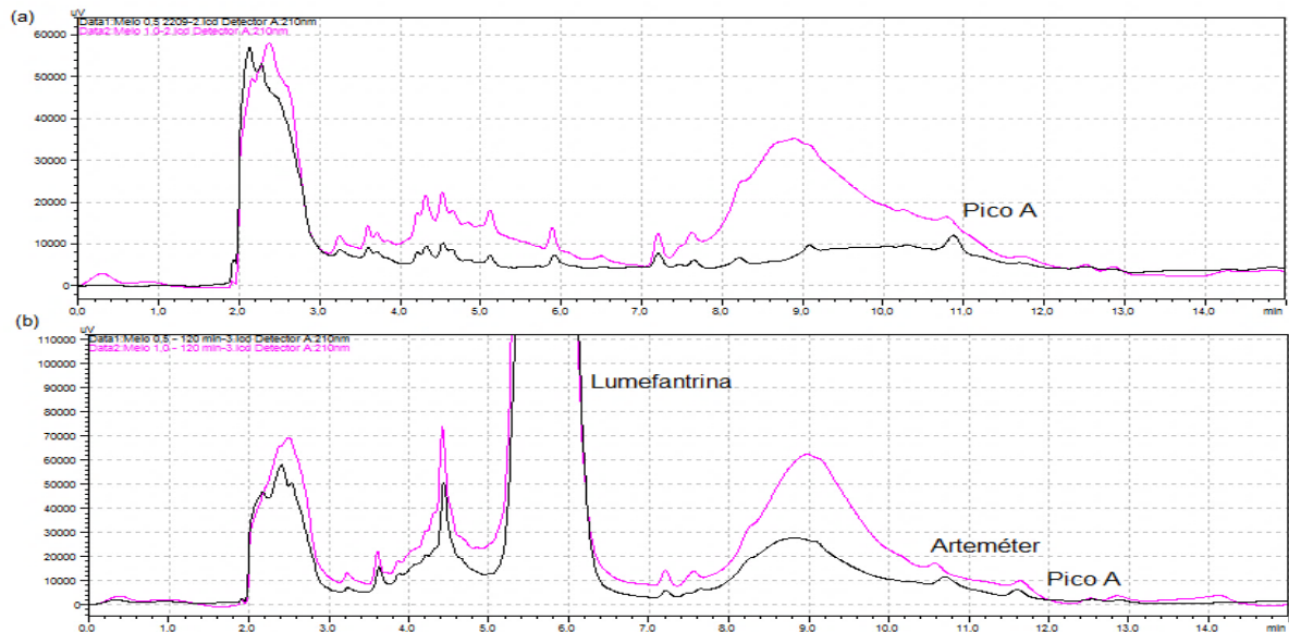
Figura 323 - Comparação dos cromatogramas para a) meios de dissolução pH 1,2 + 0,5% P80 (p/v) e pH 1,2 + 1,0% P80 (p/v); b) amostra dissolvida nos meios de dissolução pH 1,2 + 0,5% P80 (p/v) e pH 1,2 + 1,0% P80 (p/v), pás, 100 rpm
