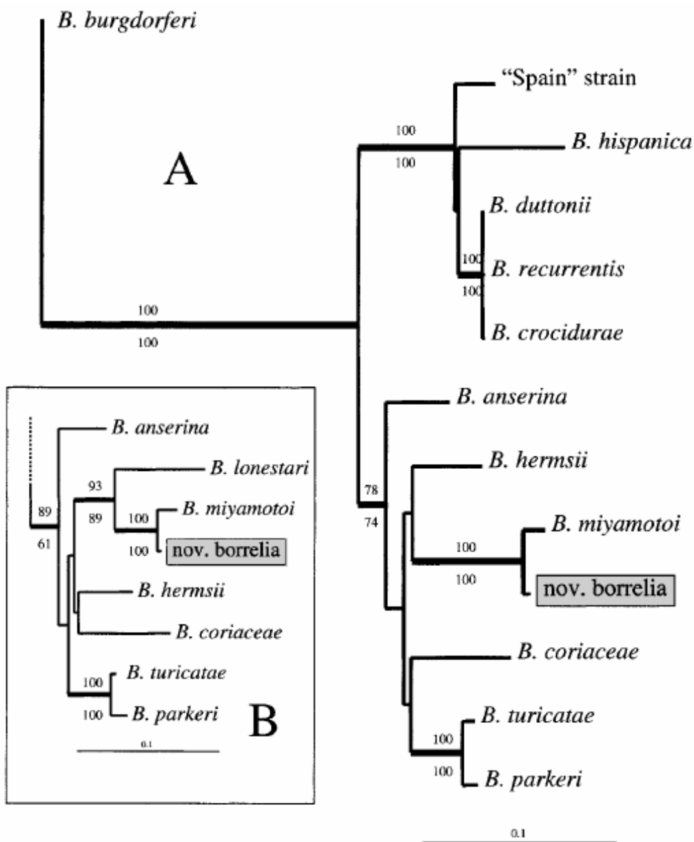
Figura 2: Árvore filogenética derivada da análise do alinhamento de seqüências do gene flagelina de 13 espécies de Borrelia (SCOLES et al., 2001).
