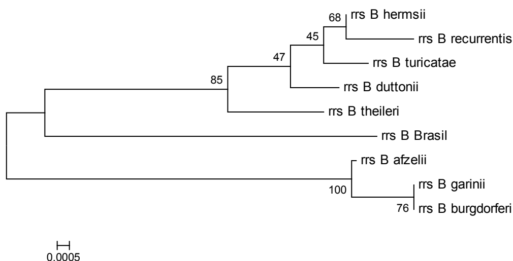
Figura 11: Árvore filogenética obtida através do método neighbor-joining contendo as seqüências de fragmentos de RRS de espécies de Borrelia do grupo B. burgdorferi e febre recorrente disponíveis no Genbank e a seqüência preditiva de aminoácidos de Borrelia isolado Brasileiro (B Brasil), amplificadas a partir do oligonucleotídeo iniciador rrs3 (112 aminoácidos) DNA proveniente de bovino sorologicamente reativo à B. burgdorferi . Os números nos nós indicam os valores de bootstrap para 1000 réplicas.
